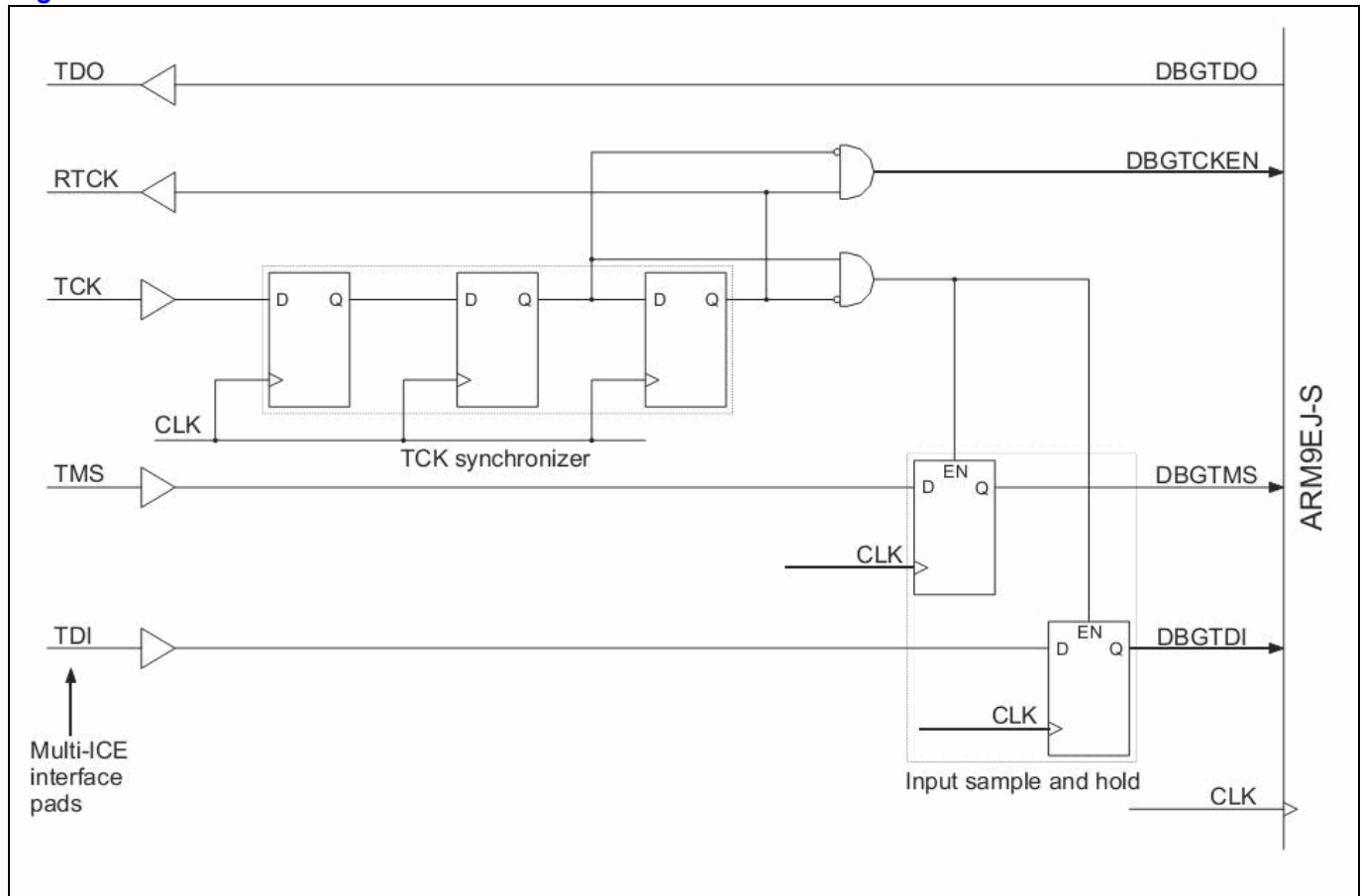
Figure 24-3 JTAG interface 회로
